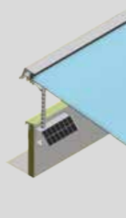
Typ L/EL-KS Kettenantrieb mit integriertem Solarpaneel und Funksteuerung für energieautarke Betätigung, Hubhöhe: bis 300 mm
