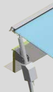
Typ L/EL-24 Spindelhubmotor für elektrische Lüftung, 24 V Gleichstrom, Hubhöhen: 300 mm oder 500 mm
