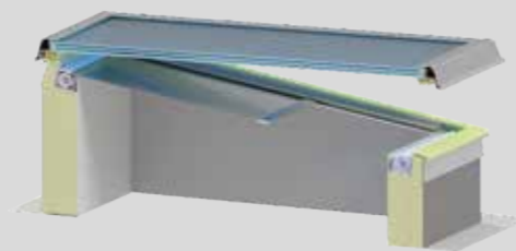
MULTIFILM® Sonnen- und Blendschutzsystem eingebaut. Ansicht Schnitt.
