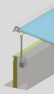
Typ L/EL-K Kettenantrieb in verdecktem Einbau, mikroprozessorgesteuerter Motor mit Kettenaustritt, Hubhöhe: bis 500 mm
