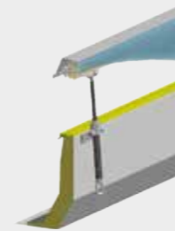
Typ L/SP Teleskopspindeltrieb mit Handkurbelstange, Hubhöhe: 300 mm
