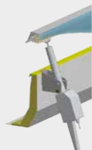
Typ L/EL-24 Elektrische Lüftung, 24 V Gleichstrom, Hubhöhen: 300 mm oder 500 mm
