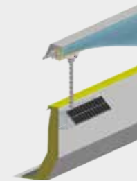
Typ L/EL-KS Kettenantrieb mit integriertem Solarpaneel und Funksteuerung für energieautarke Lichtkuppel- betätigung, Hubhöhe: bis 300 mm
