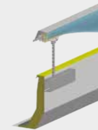
Typ L/EL-K Kettenantrieb, mikropro- zessgesteuerter Motor mit Kettenaustritt, Hubhöhe: bis 500 mm
